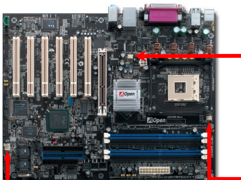
SYSFAN3 接頭
