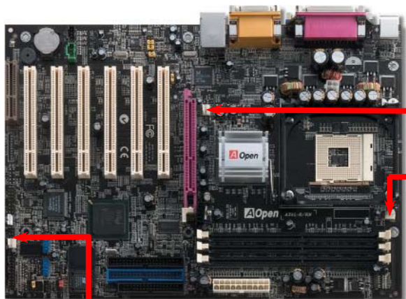
CPU 散熱風扇電源接頭
