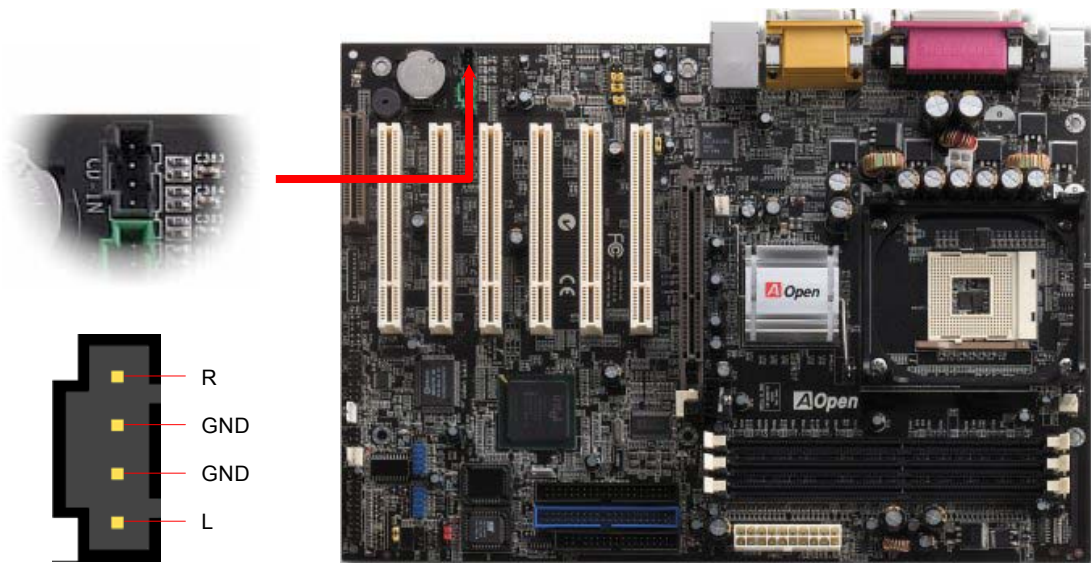
CD-IN 接頭
