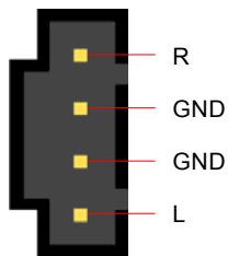
CD-IN 接頭
