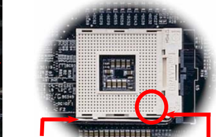
CPU 插槽固定桿
