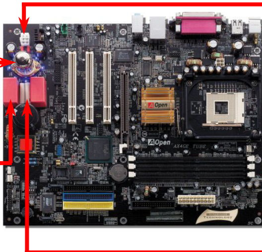
オーディオケーブルコネクタ
