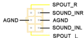
オーディオケーブルコネクタ
