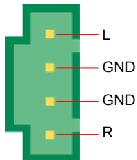
AUX-IN 接頭
