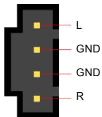
CD-IN 接頭
