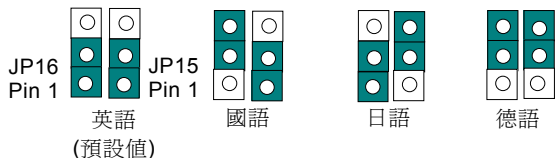
Dr. Voice II 語言選擇開關
