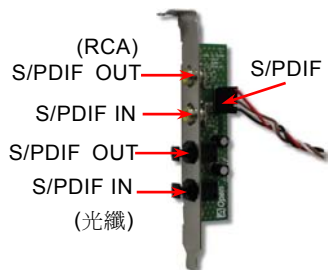
S/PDIF 模組 (用戶選配)
