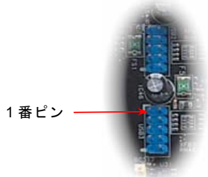
USB4 及び USB3 コネクタ
