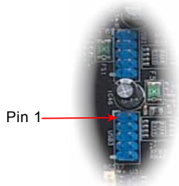
第二/第三組 USB 接頭
