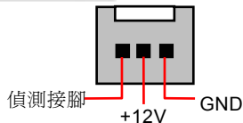
SYSFAN3 接頭
