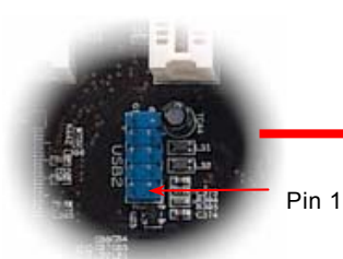
USB2 接頭
