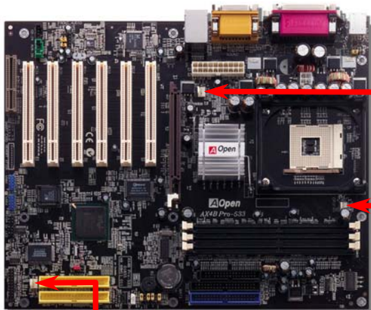
CPU ファンコネクタ
