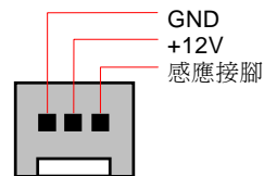
FAN2 接頭
