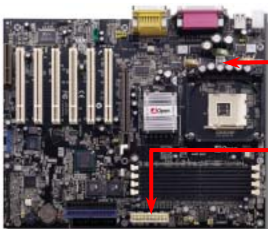
4-Pin 12V ATX 電源接頭
