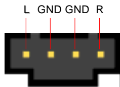
CD-IN 接頭
