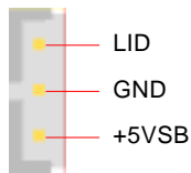
WOL 接腳
