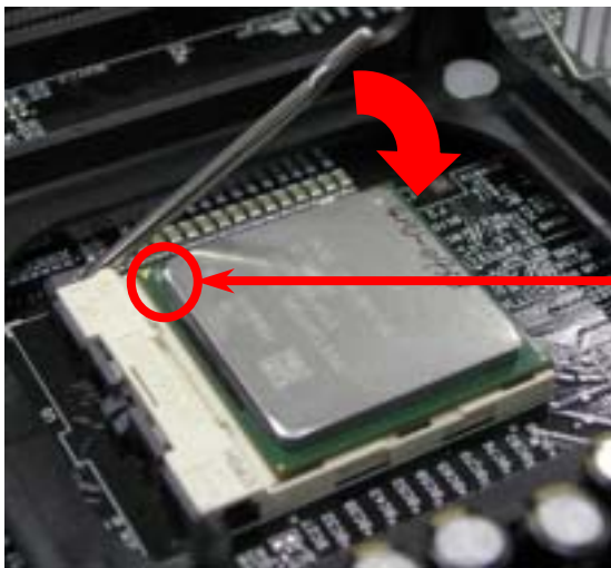
CPU 缺角
