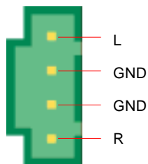
AUX-IN 接頭
