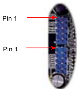
USB3 及 USB4 接頭
