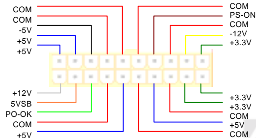
20-Pin 電源接頭
