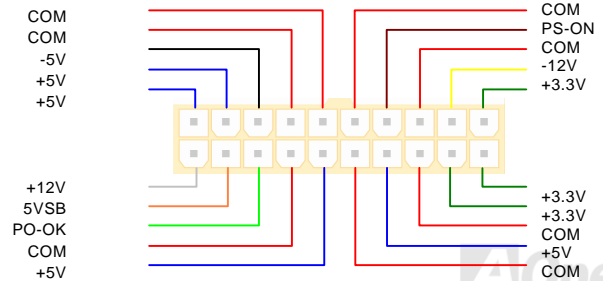
Conector de corriente 20-Pin
