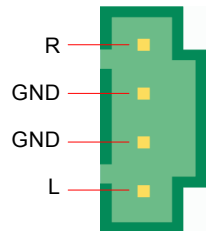
AUX-IN-Anschluss
