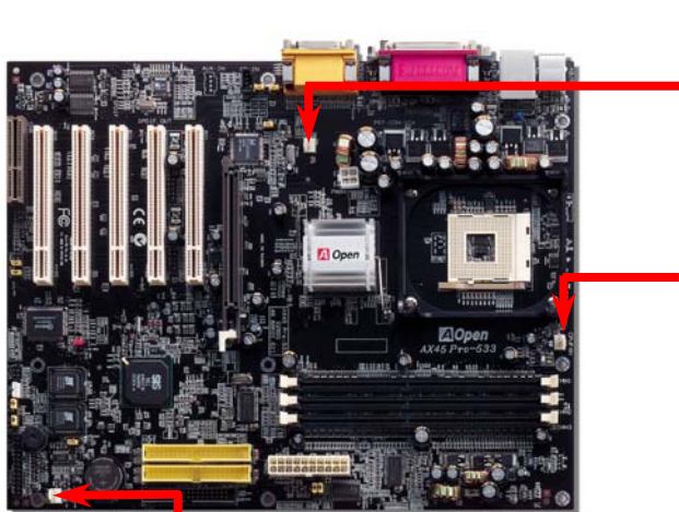
CPU FAN 接頭
