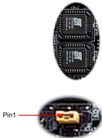
JP30 Die-Hard BIOS 選擇跳線
