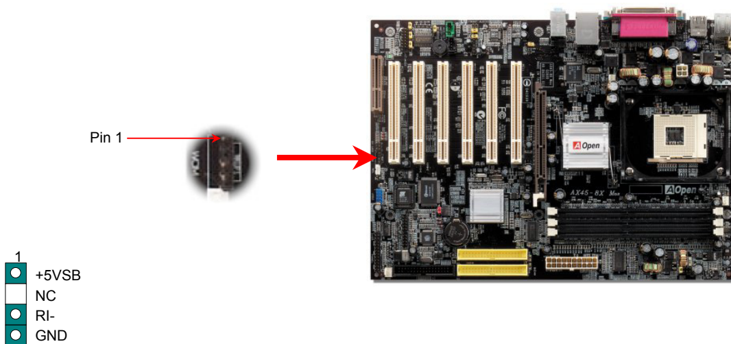
WOM 接頭
