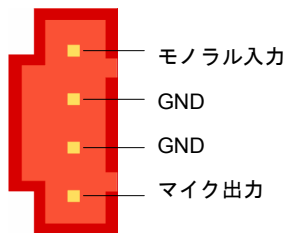
モデム入力コネクタ
