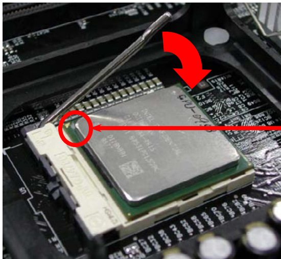
CPU-Schnittkante
