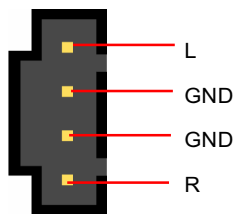
CD-IN
