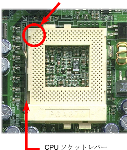
CPU の 1 番ピンと切り欠き面
