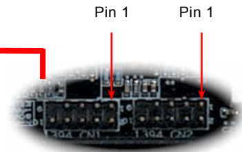
IEEE 1394 Port 1 & 2
