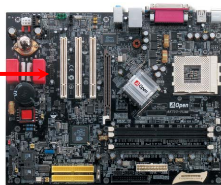
遊戲連接埠接頭
