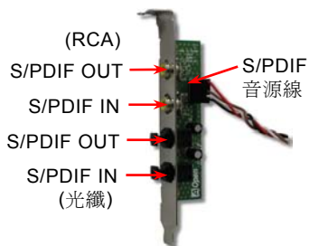
S/PDIF 模組 (用戶選配)
