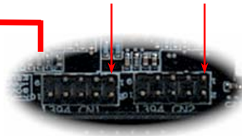
IEEE 1394 連接埠 1 & 2
