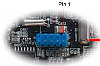
USB 2.0 接頭
