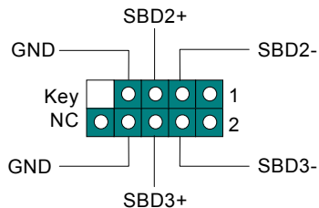
USB 2.0 接頭
