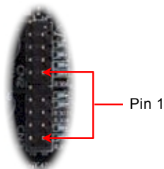
IEEE 1394 Port 1 & 2
