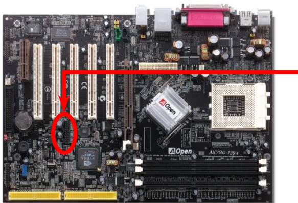
IEEE 1394 Port 1 & 2
