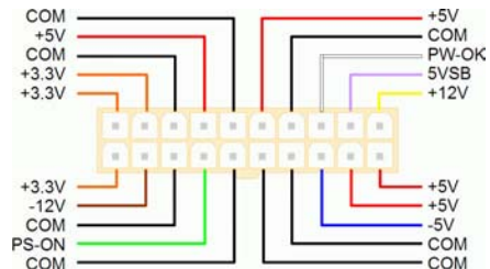
20-Pin 電源接頭
