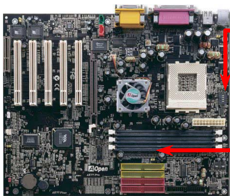
SW1 Interruptores selección relación CPU
