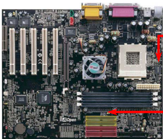
SW1 CPU レシオ 設定スイッチ
