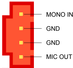
MODEM-CN-Anschluss
