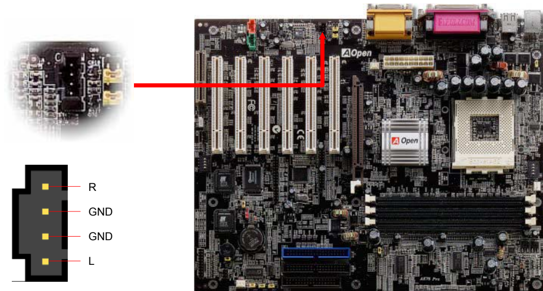
CD-IN-Anschluss
