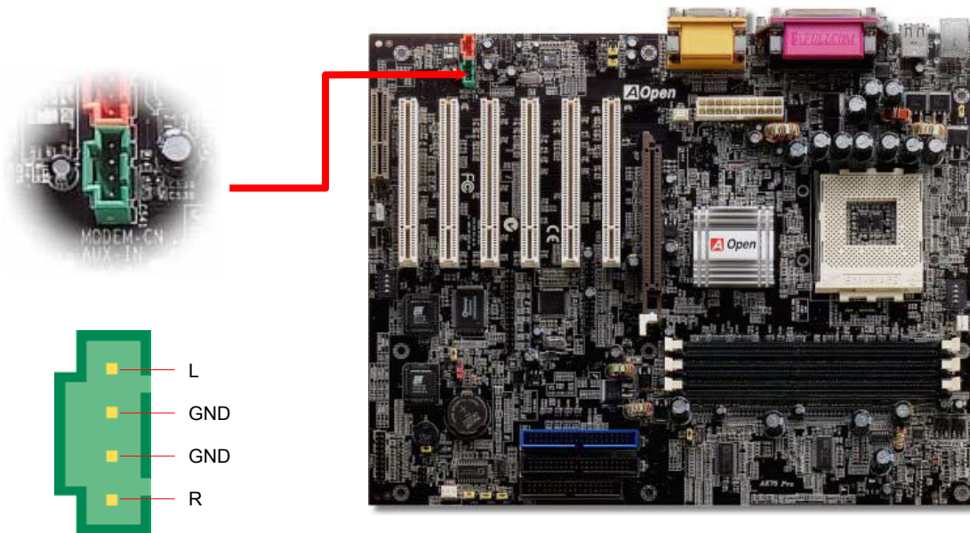
AUX-IN-Anschluss
