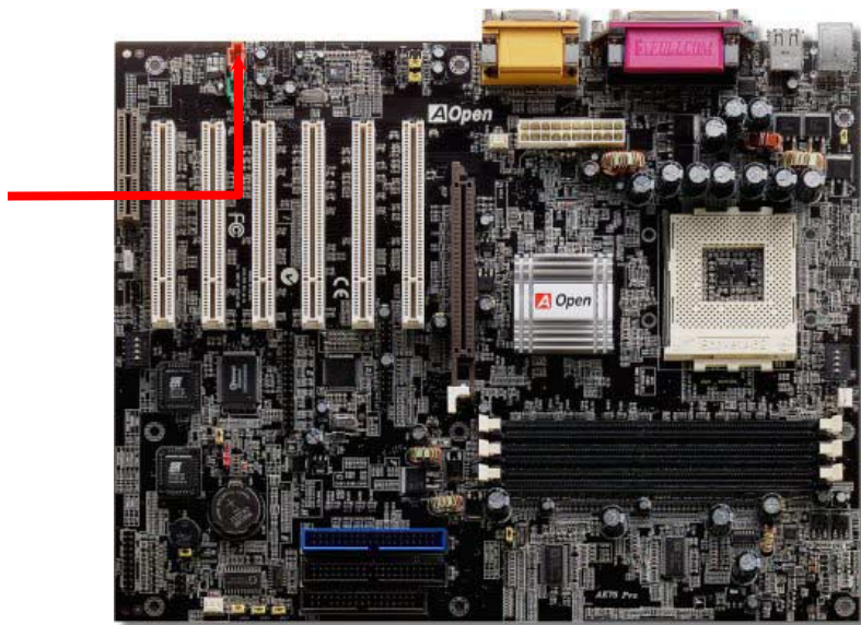
MODEM-CN 數據機音源接頭
