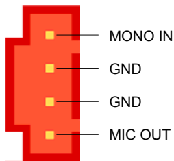
MODEM-CN 數據機音源接頭
