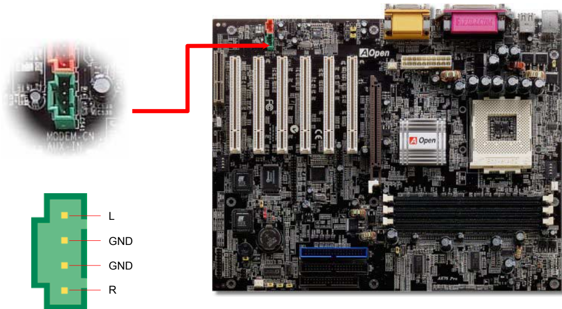
AUX-IN 外接音源輸入接頭
