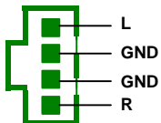
VIDEO_AUDIO_IN
