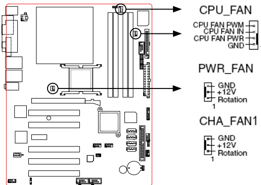
Fan connectors
