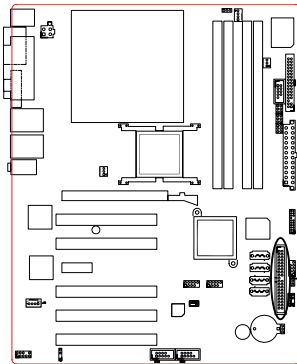
IDE connector
