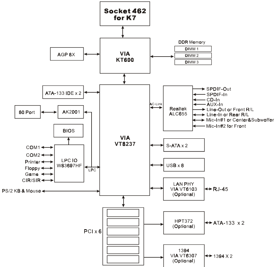
<图5> 系统方块图
