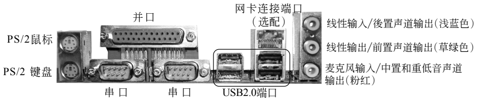
<图3> 输入/出连接端口
