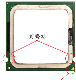
黃色三角標記即為 Pin 1 指示器
