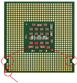
黃色三角標記即為 Pin 1 指示器
