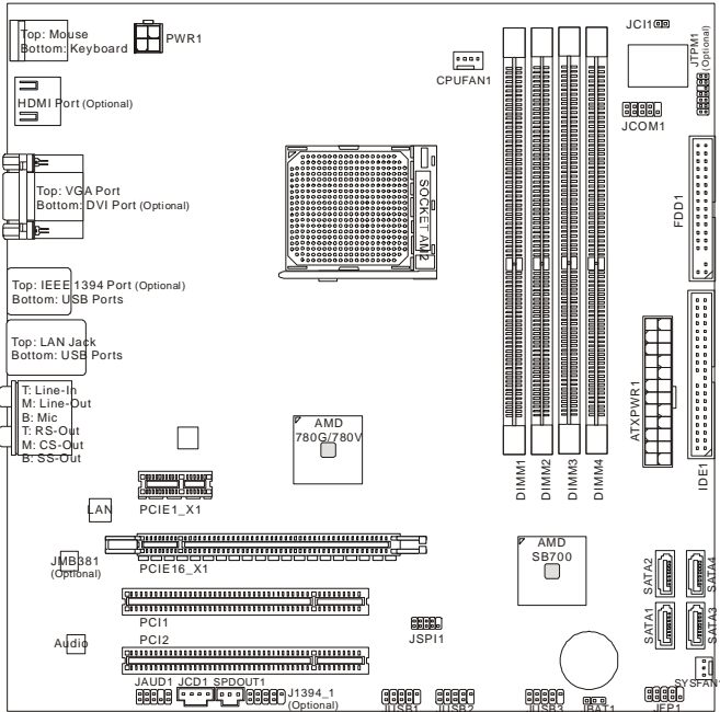
K9A2GM / K9A2VM (MS-7501 v1.X) Micro-ATX Mainboard
