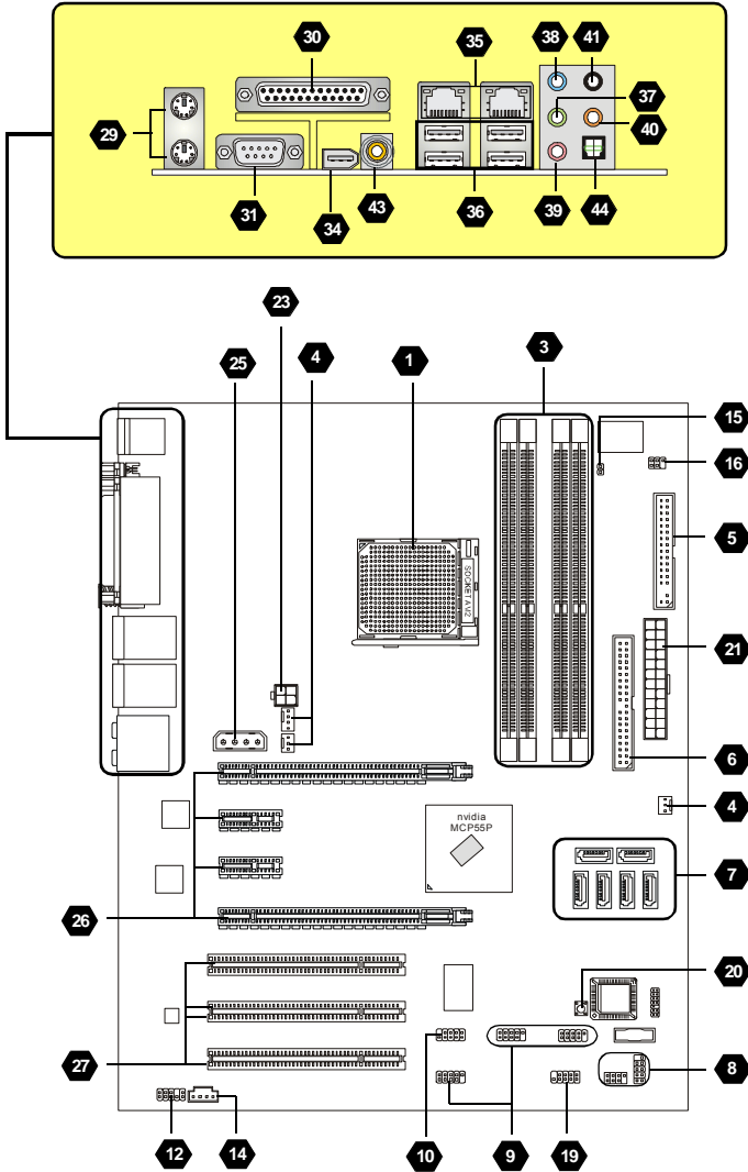
Carte Mère K9N SLI Platinum Séries (MS-7250 v1.X)
