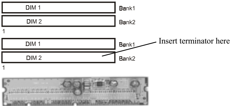
DDR Terminator module
