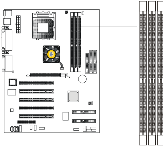
DDR DIMM Slots (DIMM 1~3)
